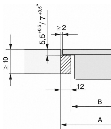
CS 7000 FL, à fleur de plan (schéma)
